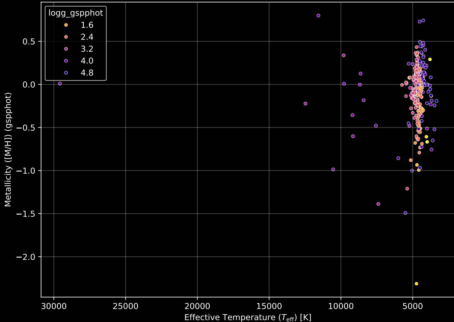
APOGEE DR17 Field: [140-18_btx] Stellar Population Parameters (n= 310)
